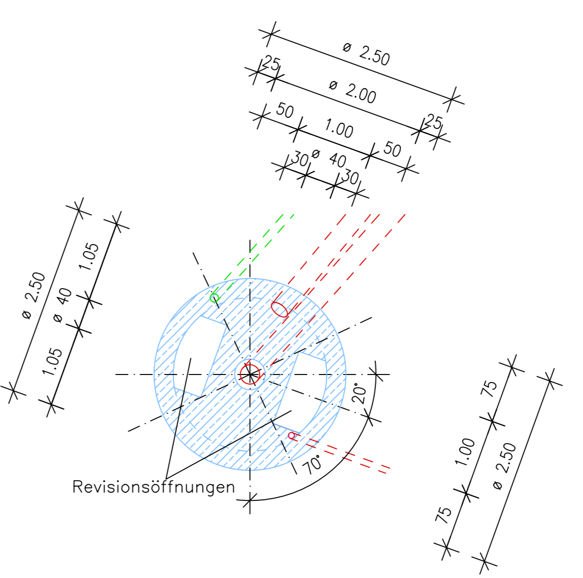
Schnitt 1-1 Maßstab 1:50
