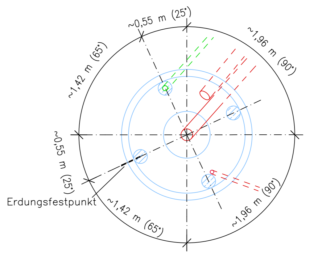
Schnitt 3-3 Maßstab 1:50
