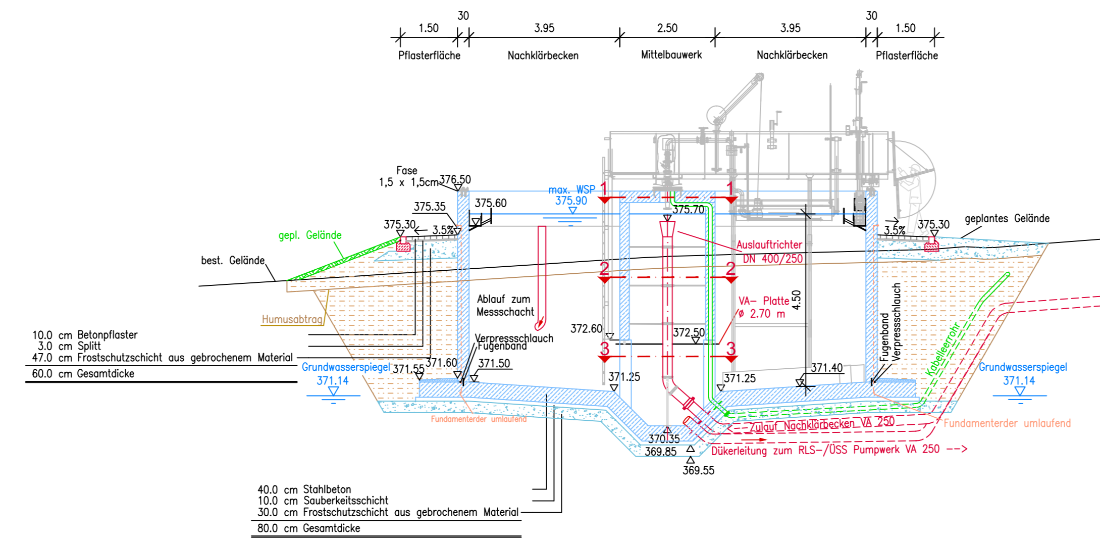
geplantes Nachklärbecken Schnitt A-A
