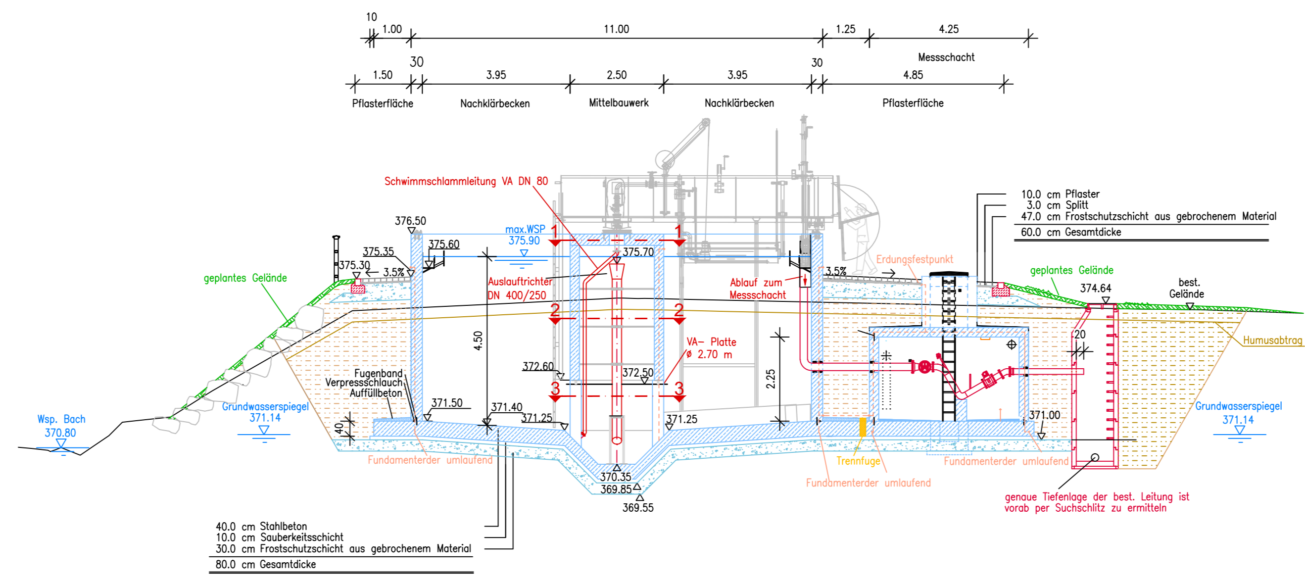
geplantes Nachklärbecken Schnitt B-B
