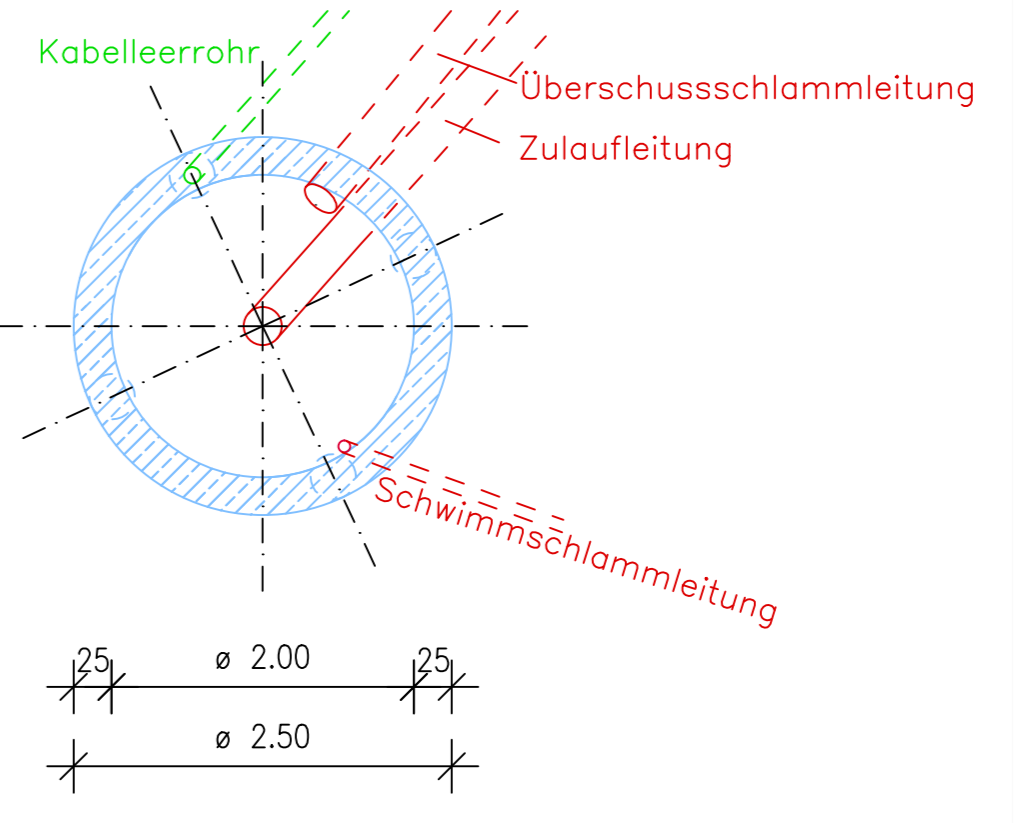
Schnitt 3-3 Maßstab 1:50
